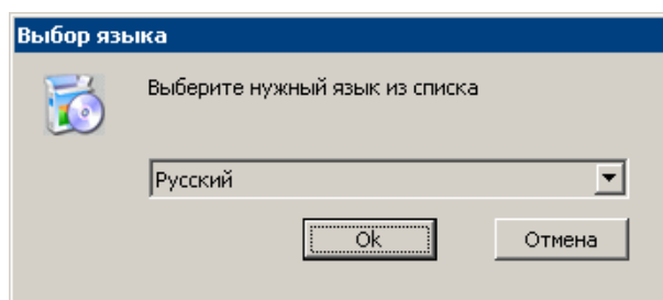
Рис. 2.11. Выбор языка
